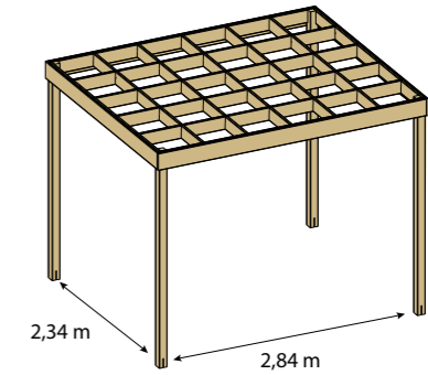
ESTEREL 3x2,5 Longueur: 3m Profondeur: 2,5m Hauteur: 2,4m Réf: 615000615
