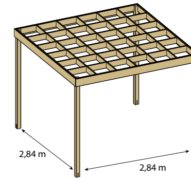
ESTEREL 3x3 Longueur: 3m Profondeur: 3m Hauteur: 2,4m Réf: 615000616
