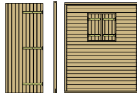
kit 1 portes + panneau fenêtre Livré avec serrure Fermeture du volet (600 x 600mm) par crochet Réf. 610000315
