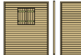
kit panneau fenêtre + panneau 905mm Fermeture du volet (600 x 600 mm) par crochet Réf. 610000316
