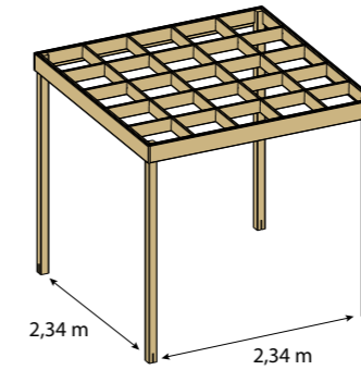
ESTEREL 2,5x2,5 Longueur: 2,5m Profondeur: 2,5m Hauteur: 2,4m Réf: 615000614
